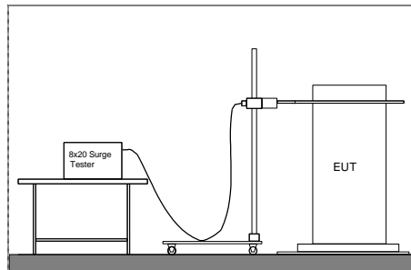
EUT setup
